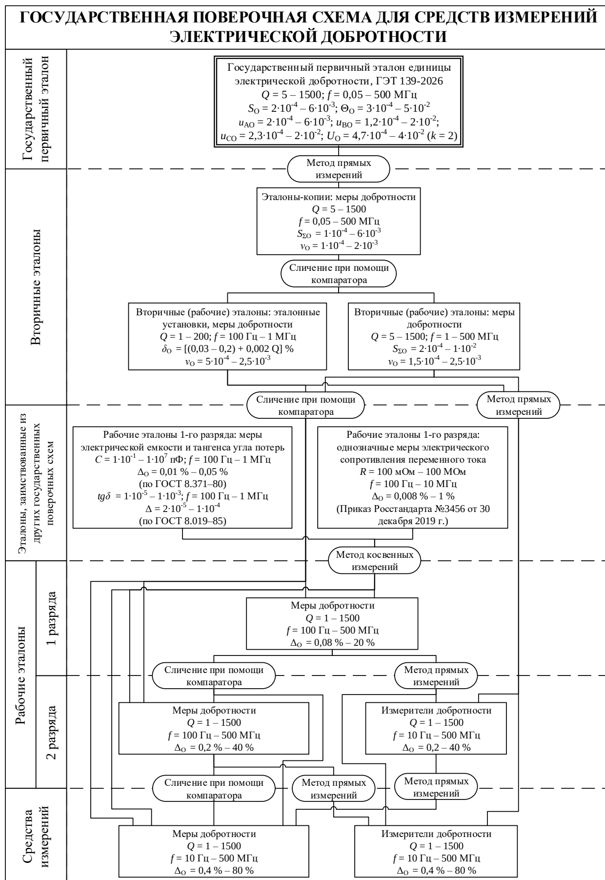
Рисунок А.1 - Государственная поверочная схема для средств измерений электрической добротности
