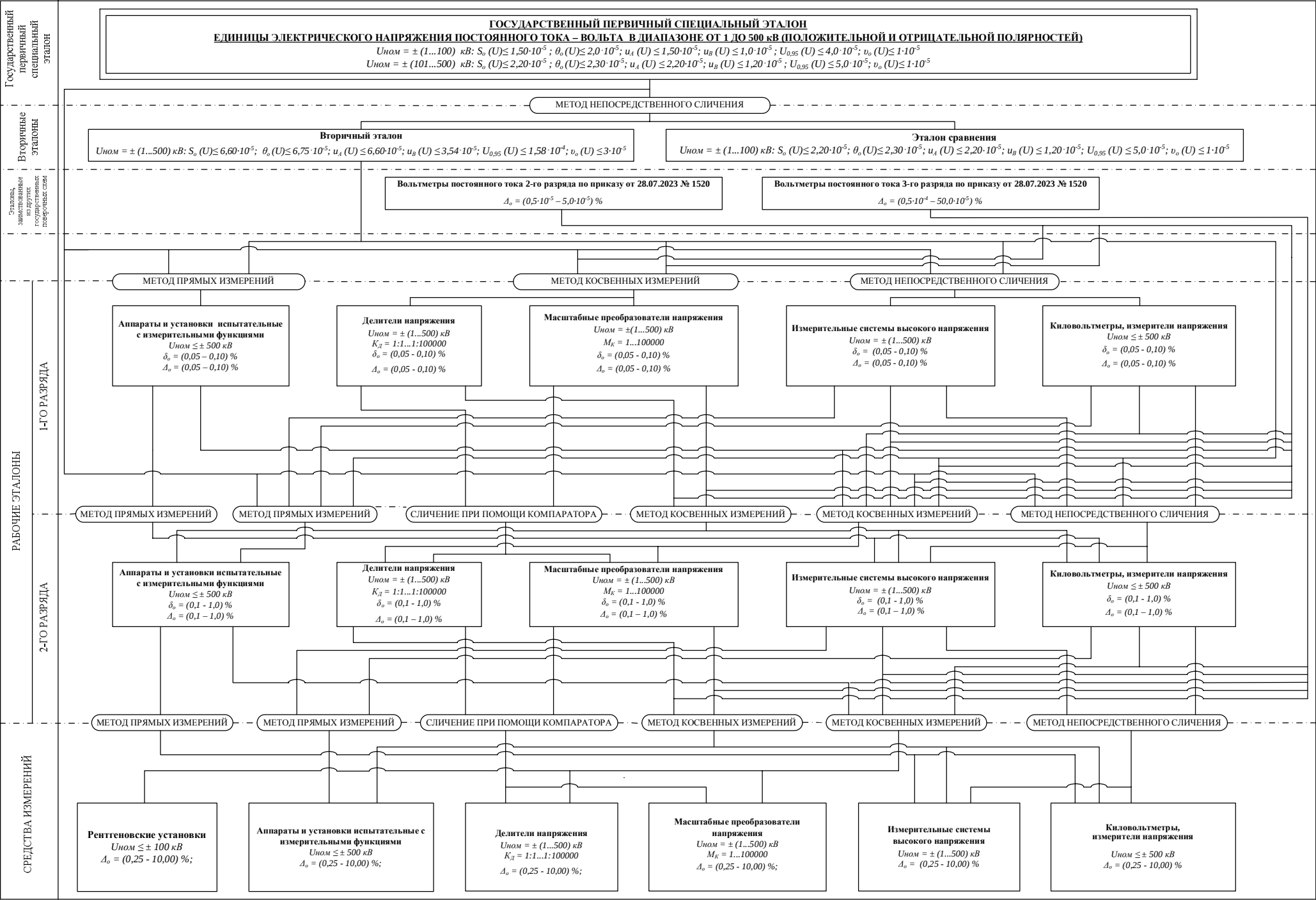
Государственная поверочная схема для средств измерений постоянного электрического напряжения в диапазоне от 1 до 500 кВ (положительной и отрицательной полярностей)
