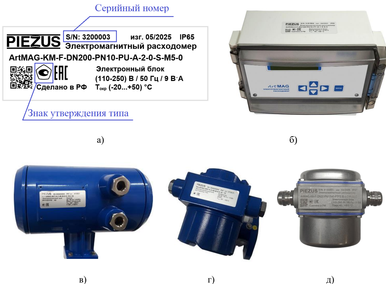
Рисунок 5 – Вид маркировочной этикетки электронного блока и места ее нанесения на электронные блоки различного исполнения:
