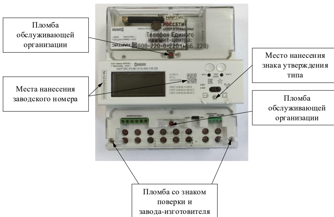
б) счетчики шкафного исполнения НАРТИС-РЗ-М
