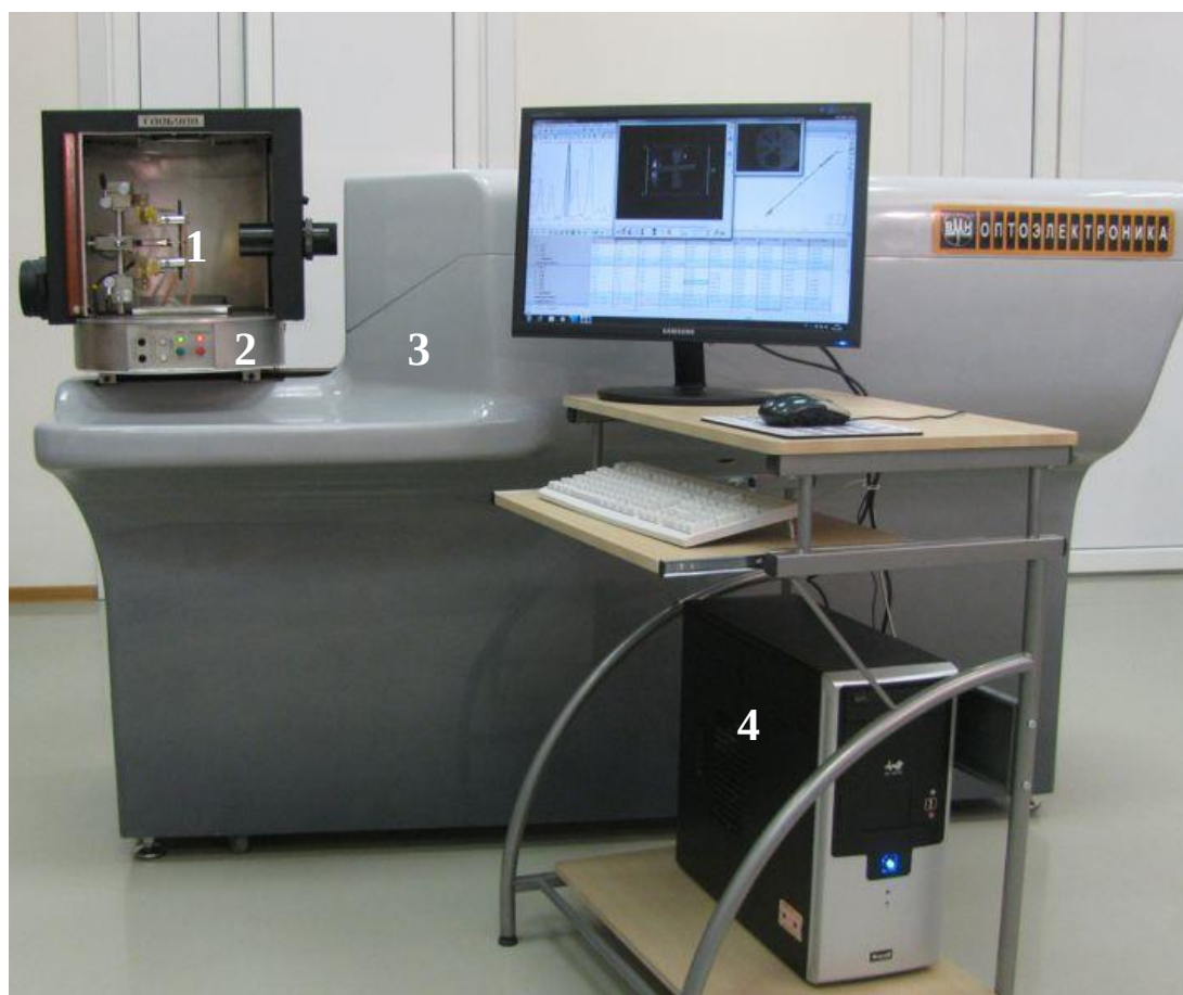
Рисунок 2 – Пример комплекса МАЭС на базе спектрального прибора с дуговым возбуждением спектров 1 – исследуемый образец, 2 – источник возбуждения спектров, 3 - система разделения спектральных линий (спектрометр Гранд) с анализатором МАЭС, 4- компьютер
