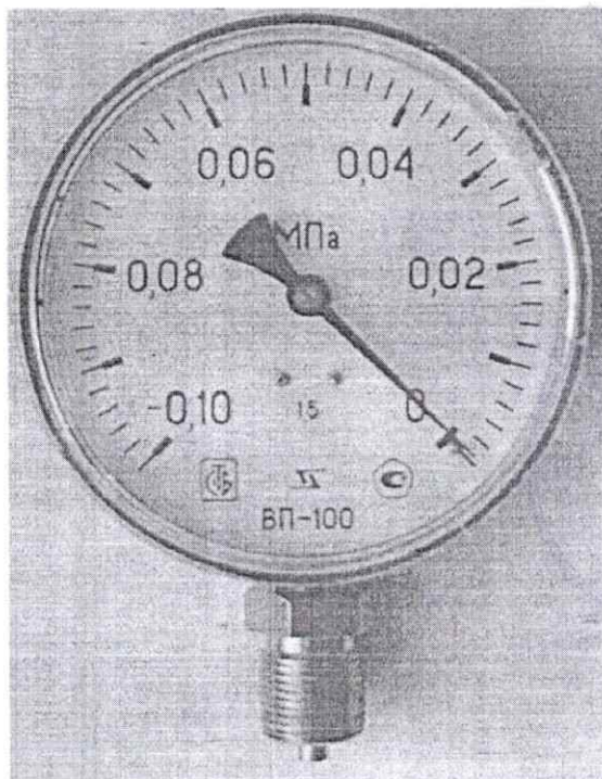
Вакуумметр показывающий ВП-100
