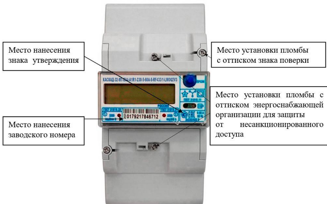
Рисунок 6 – Общий вид счетчика в корпусе типа D34
