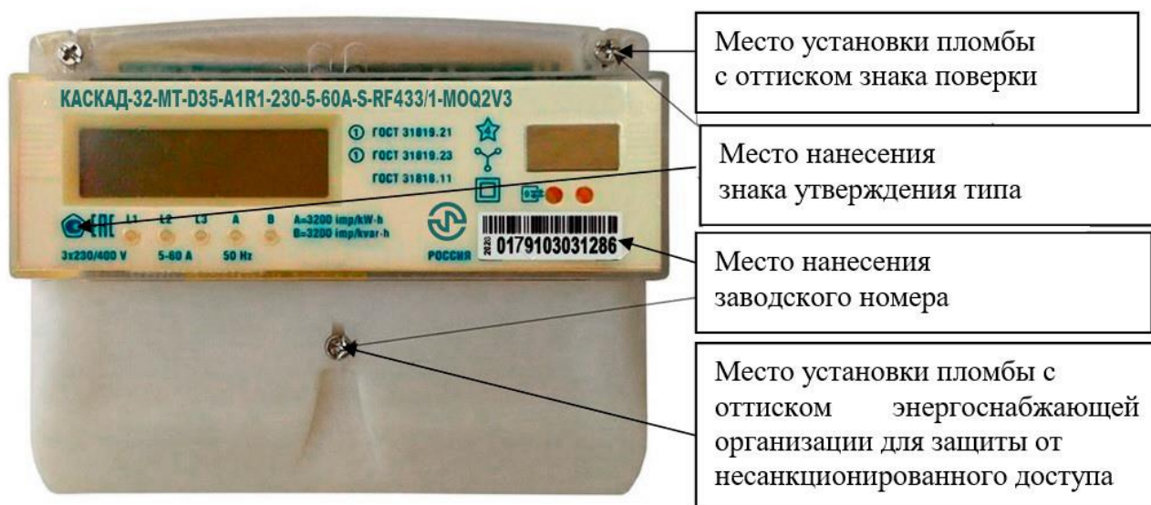
Рисунок 7 – Общий вид счетчика в корпусе типа D35
