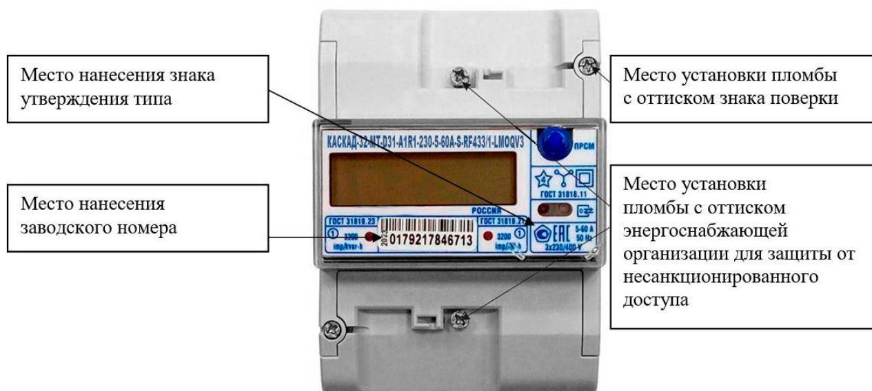
Рисунок 4 – Общий вид счетчика в корпусе типа D31
