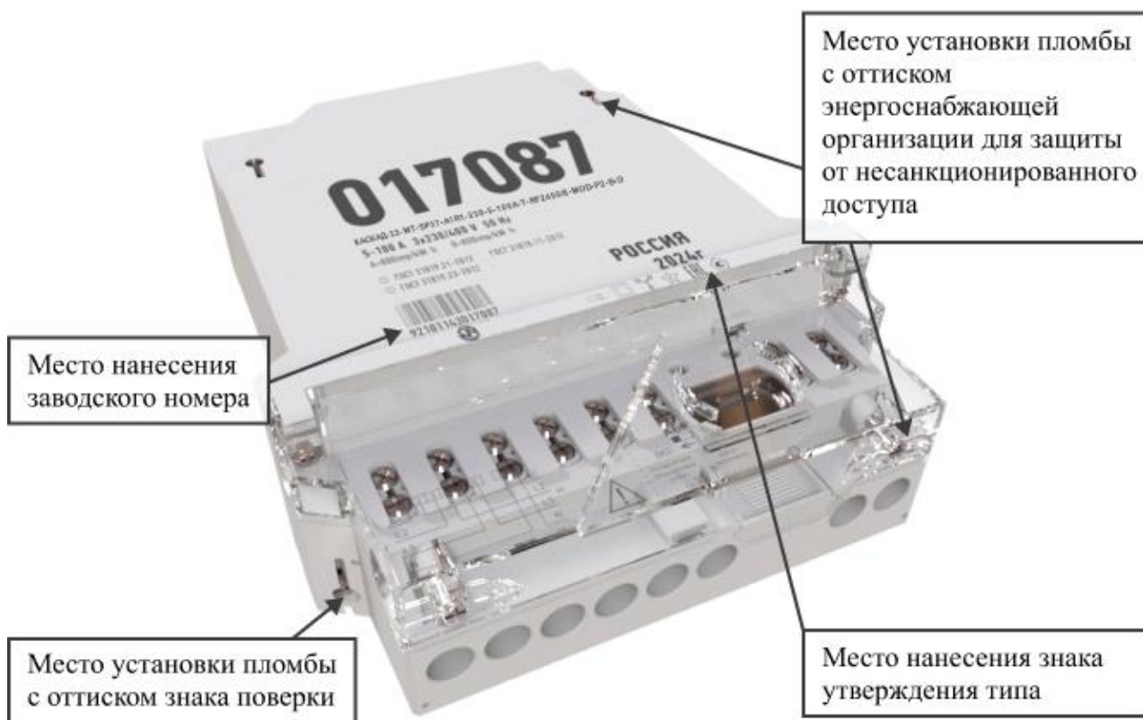
Рисунок 10 – Общий вид счетчика в корпусе типа SP37
