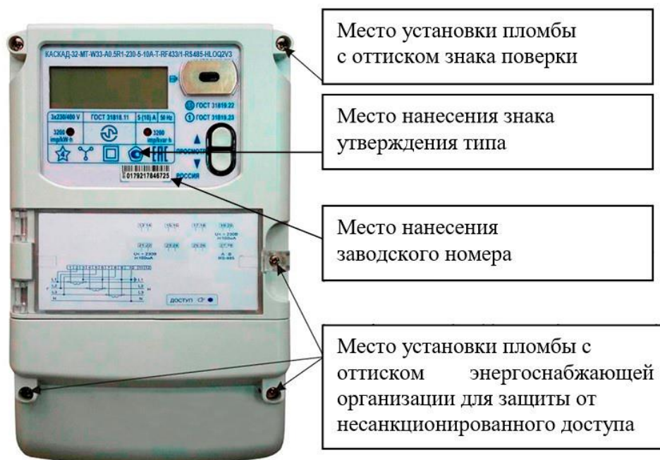
Рисунок 3 – Общий вид счетчика в корпусе типа W33
