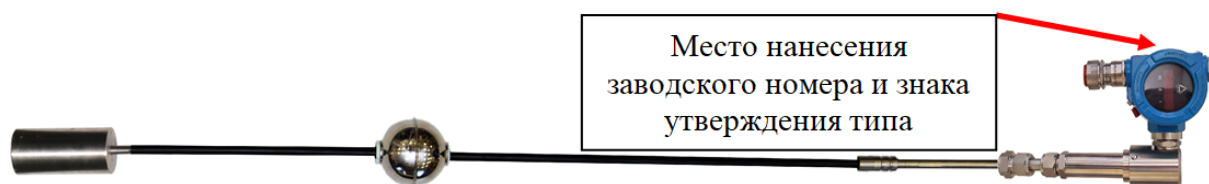
Р и с у н о к 2 – Уровнемеры ВЕКТОР21XXX-0-X-0, ВЕКТОР22XXX-0-X-0, ВЕКТОР23XXX-0-X-0, ВЕКТОР21XXX-ДТ-X-0, ВЕКТОР22XXX-ДТ-X-0, ВЕКТОР23XXX-ДТ-X-0 с гибким измерительным элементом
