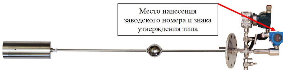
Р и с у н о к 3 – Уровнемеры ВЕКТОР10XXX-ДПТ-X-0, ВЕКТОР11XXX-ДПТ-X-0 с жестким измерительным элементом
