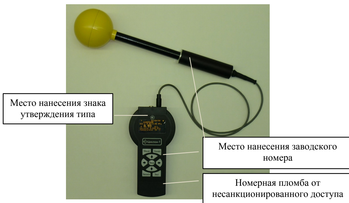
А) Блок измерительный «Циклон-Т» с антенной АЭ1
