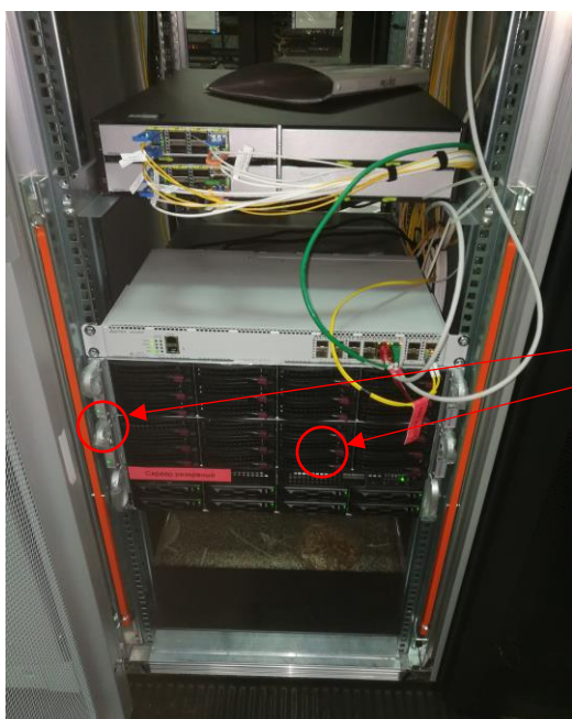
Рисунок 2 – Внешний вид сервера Системы КМУТ, установленного в статив Место нанесения знака утверждения типа
