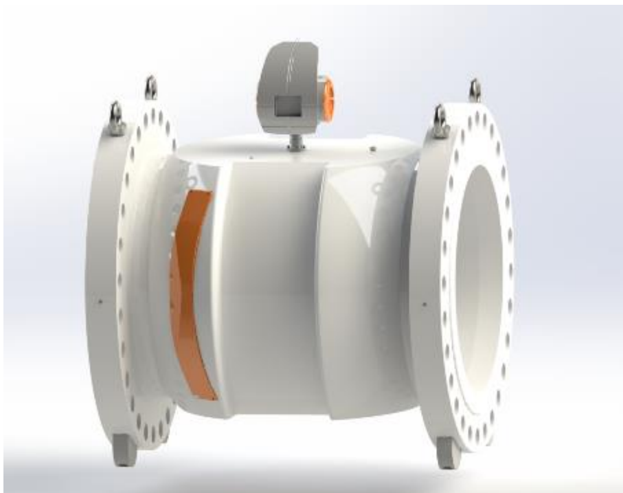
Рисунок 1 – Внешний вид счетчика модификации КТМ700 РУС Н
