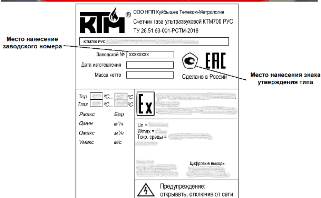
Рисунок 8 – Маркировочная табличка счетчика модификации с БОИ-Лайт
