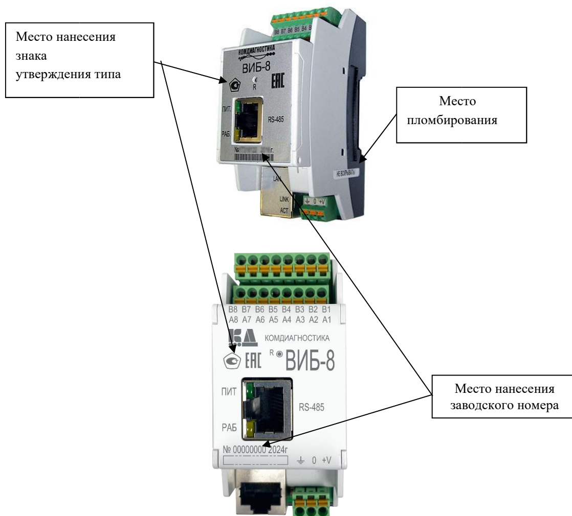
Рисунок 1 – Общий вид, место нанесения знака утверждения типа, место нанесения заводского номера и место пломбирования приборов для измерения параметров вибрации многоканальных ВИБ-8
