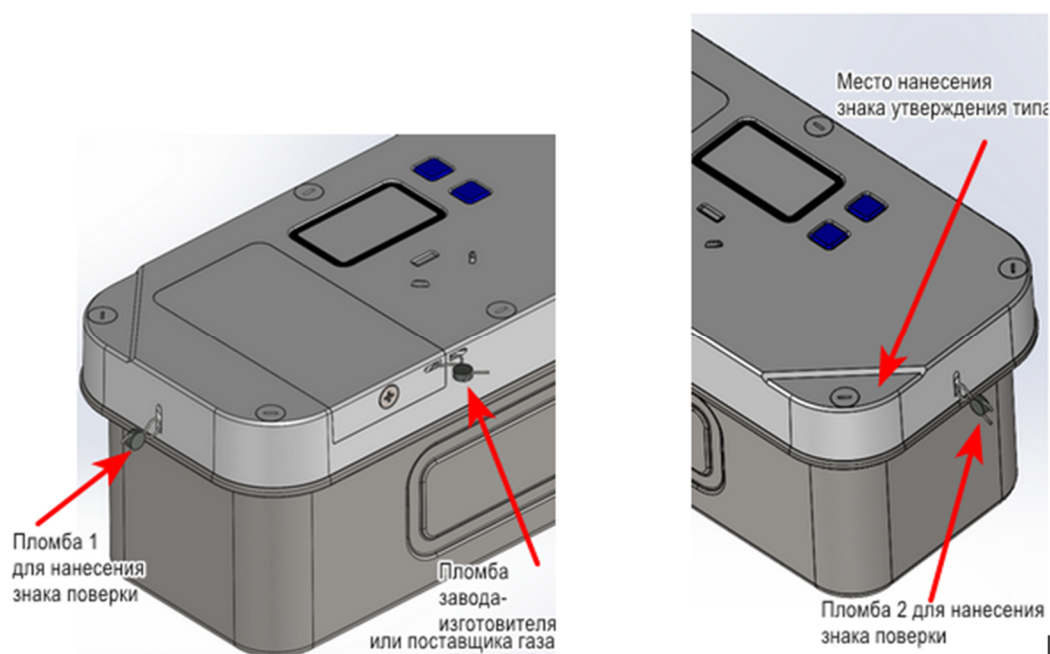
Рисунок 2 – Схема пломбировки от несанкционированного доступа, обозначение мест нанесения знака поверки, пломбы изготовителя или поставщика газа и знака утверждения типа
