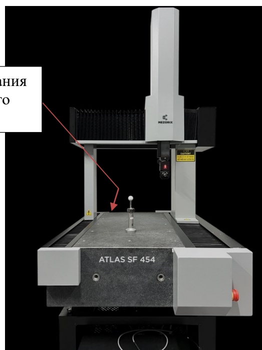
Рисунок 2 – Общий вид машин координатных измерительных MEZORIX модификации ATLAS SF
