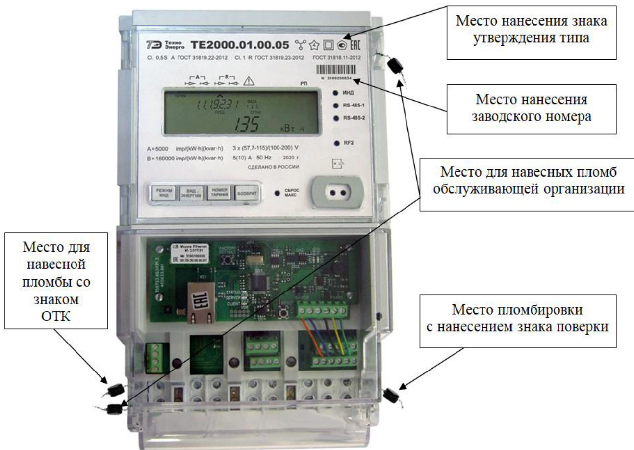
Рисунок 1 – Общий вид счетчика внутренней установки с указанием мест пломбировки от несанкционированного доступа, мест нанесения знака утверждения типа, знака поверки, заводского номера
