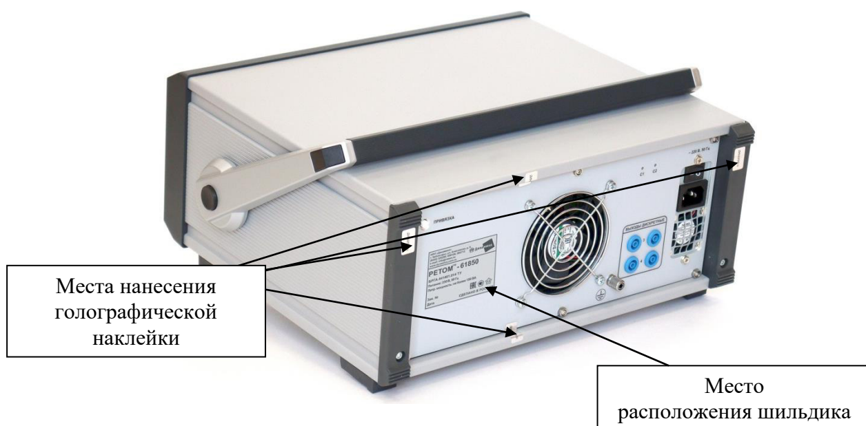
б) вид сзади с указанием мест пломбирования от несанкционированного доступа и места расположения шильдика
