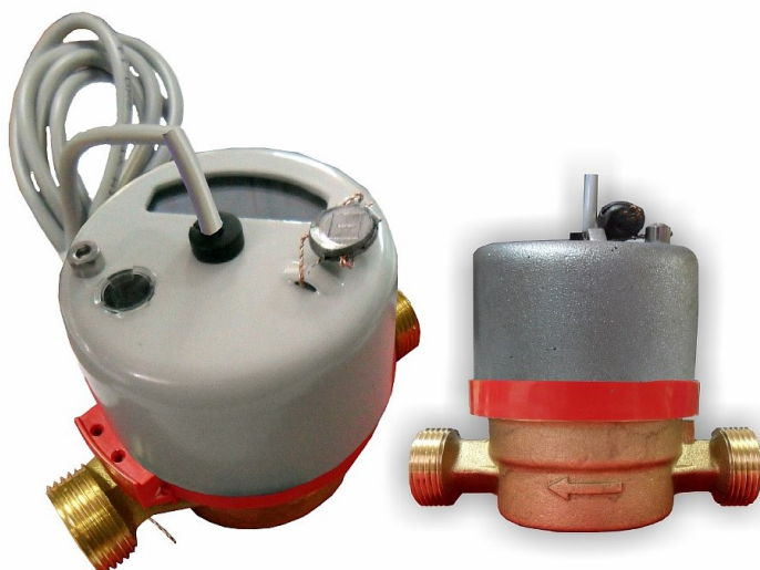
в) внешний вид счётчиков исполнений ВСТ-15, ВСТ-20, на примере ВСТ-15
