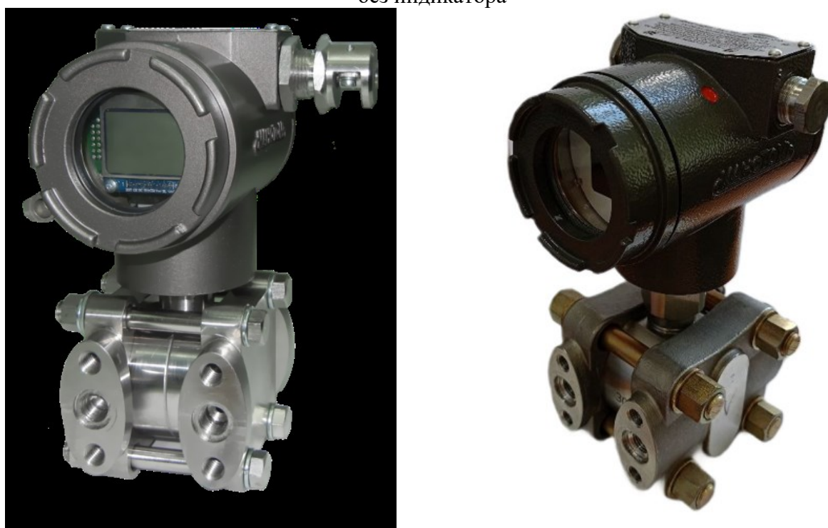
Рисунок 2 – Фотографии общего вида датчиков давления ДМ5017 фланцевого исполнения с индикатором
