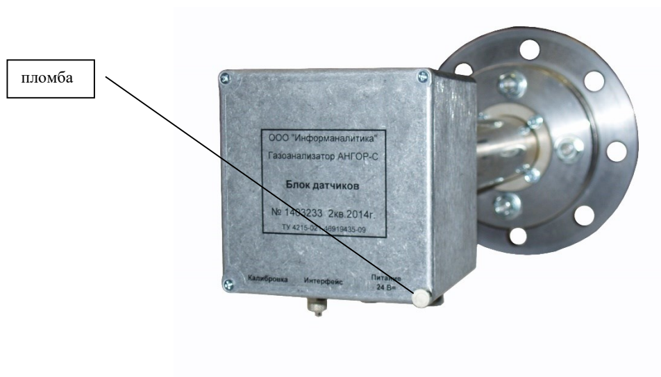
Рисунок 2 – Схема пломбировки газоанализатора
