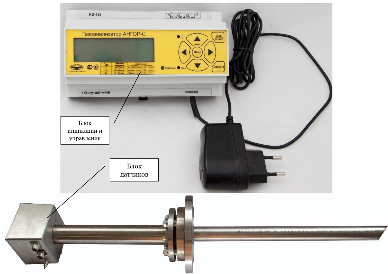
Рисунок 1 – Внешний вид газоанализатора
