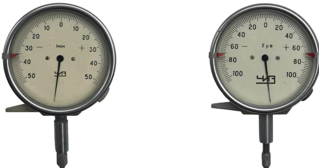
Рисунок 9 – Общий вид съемных отсчетных устройств модификации ИГ
