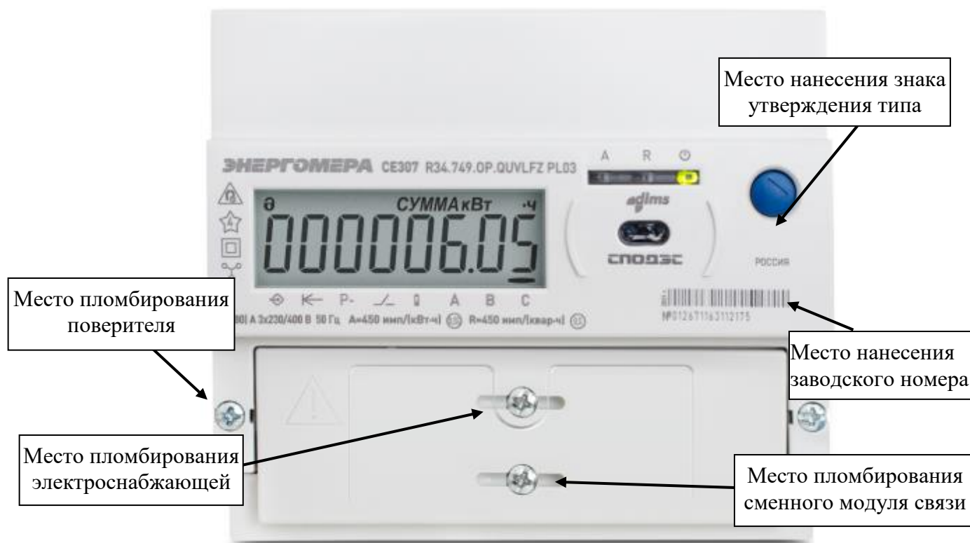
Рисунок 12 – Общий вид счетчика CE307 R34 со сменным модулем связи*
