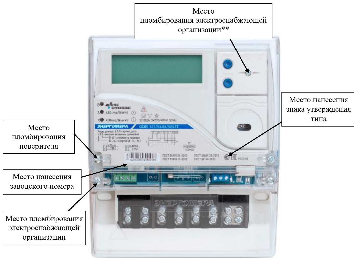
Рисунок 4 – Общий вид счетчика CE307 S31*
