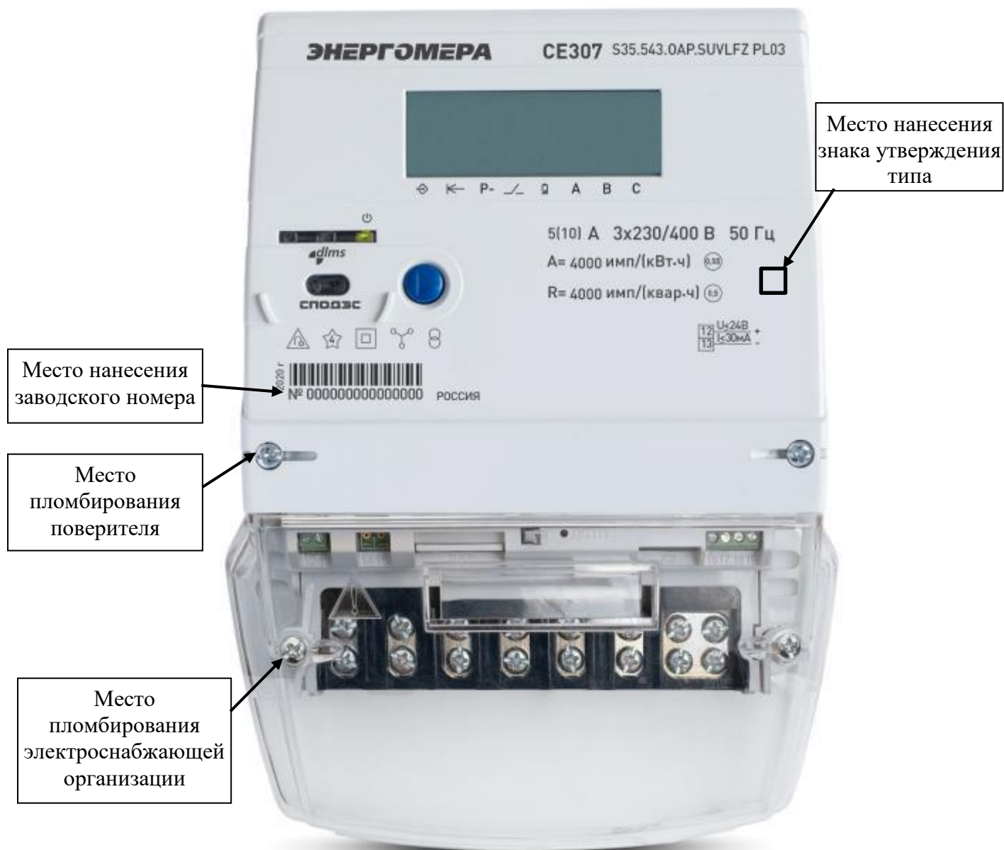
Рисунок 7 – Общий вид счетчика CE307 S35 исполнение 2*
