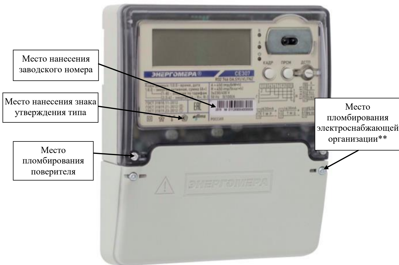
Рисунок 2 – Общий вид счетчика CE307 R32
