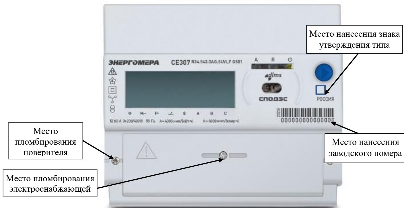
Рисунок 11 – Общий вид счетчика CE307 R34*
