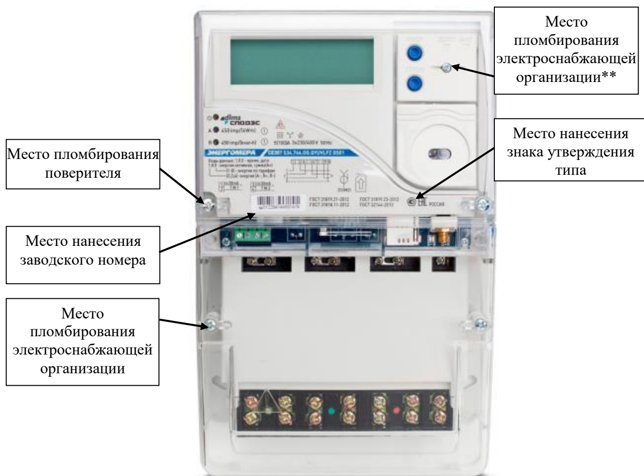
Рисунок 5 – Общий вид счетчика CE307 S34*
