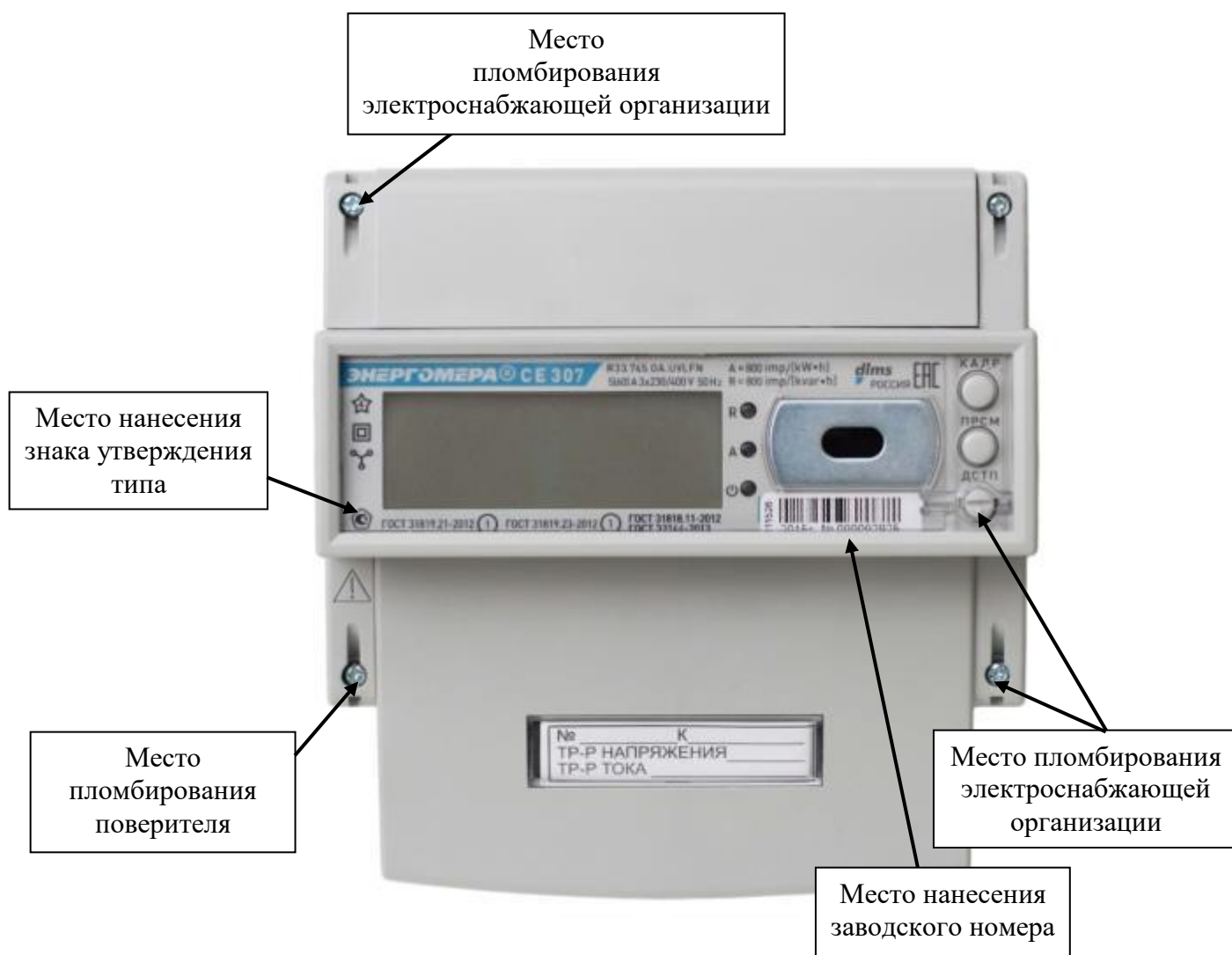
Рисунок 3 – Общий вид счетчика СЕ307 R33*
