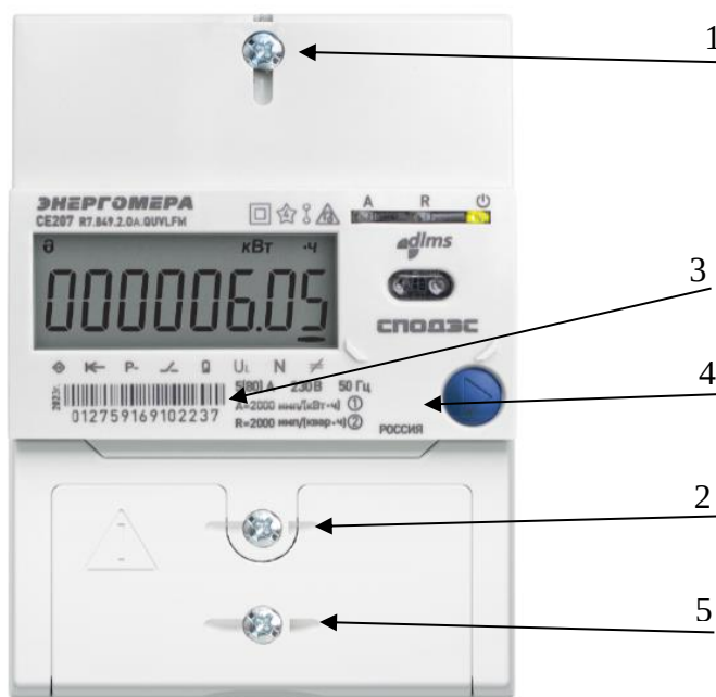
Рисунок 5 – Общий вид счетчика CE207 R7 с отсеком сменного модуля
