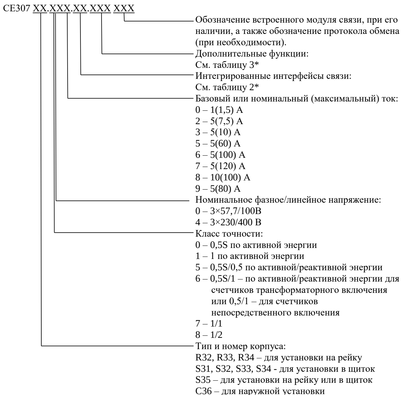
Рисунок 1 – Структура условного обозначения счетчиков
