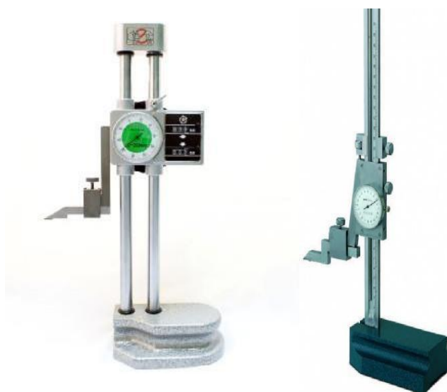
а) - Штангенрейсмас ШПК (вид 1)
