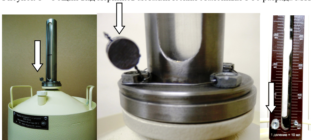
Рисунок 1 - Общий вид мерников металлических эталонных 1-го разряда М1Р
