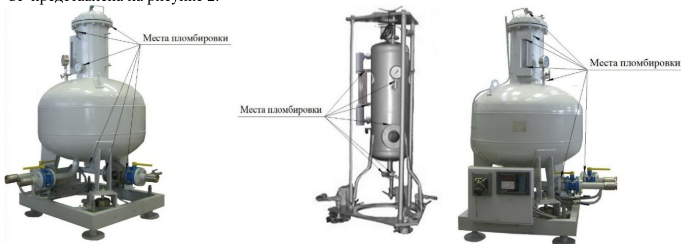
Рисунок 2 – Схема пломбировки от несанкционированного доступа, обозначение мест нанесения знака поверки установок поверочных средств измерений объема или массы сжиженных углеводородных газов УПМ-СГ
