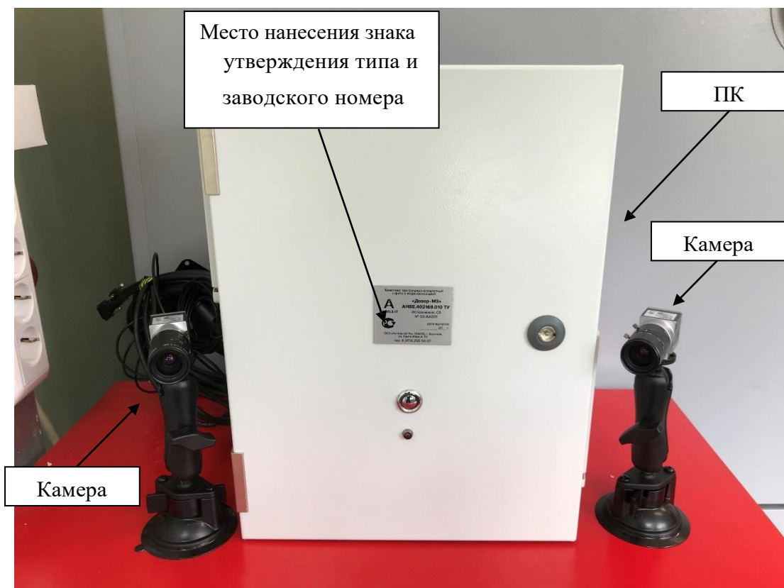
Рисунок 4 – Общий вид комплексов исполнения 03 и обозначение места нанесения знака утверждения типа и заводского номера
