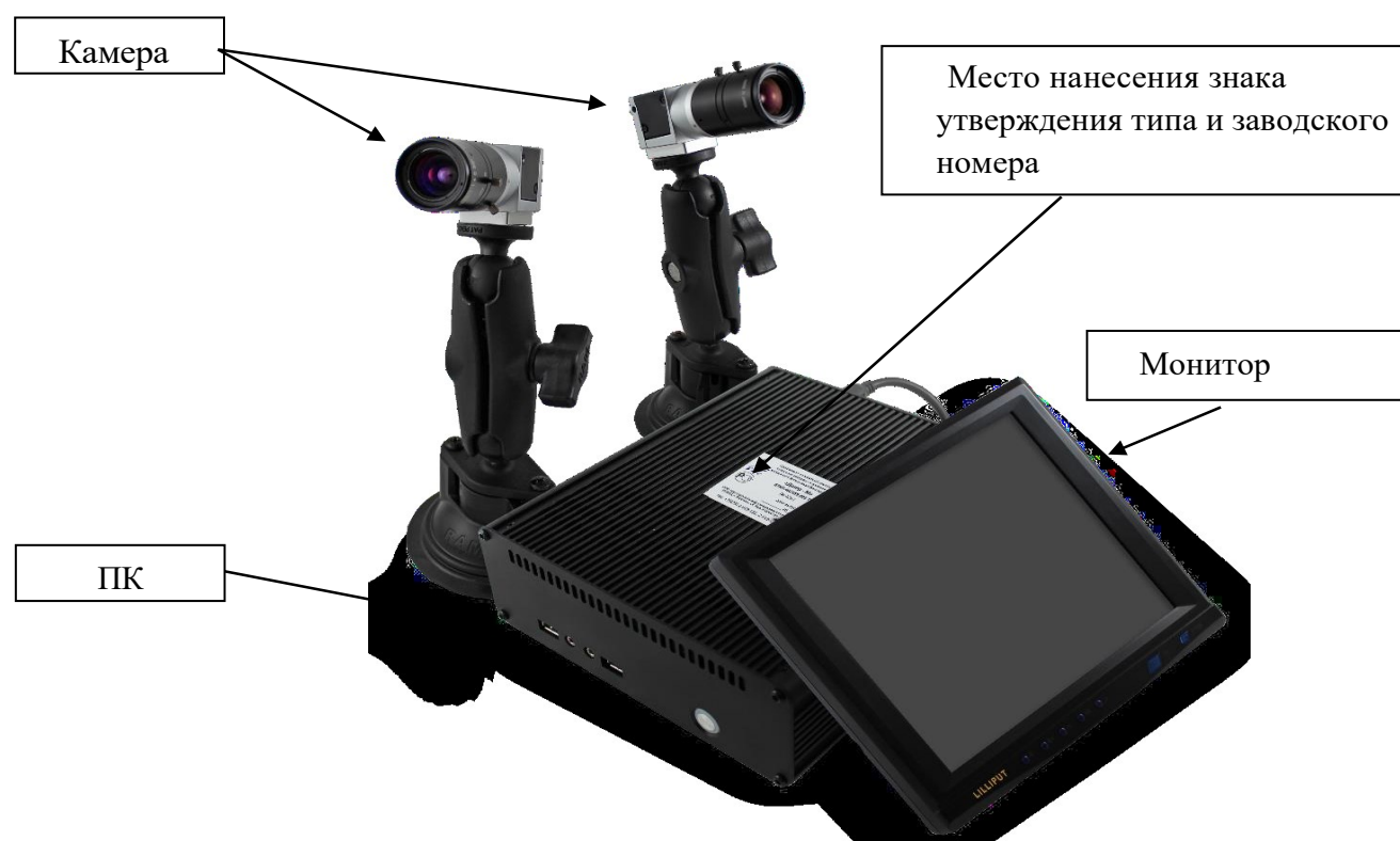
Рисунок 1 – Общий вид комплексов исполнения 01 и обозначение места нанесения знака утверждения типа и заводского номера
