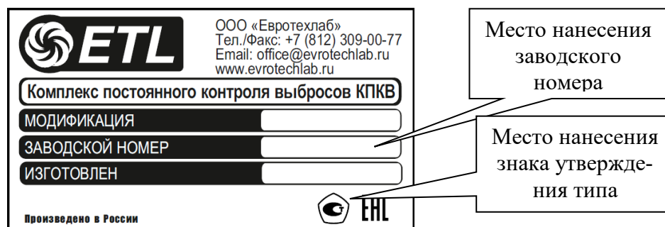
Рисунок 6 – Общий вид маркировочной таблички
