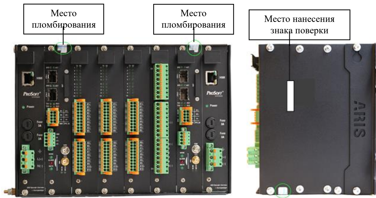
Рисунок 1 – Общий вид контроллеров исполнения ARIS-4208 с местами нанесения знака поверки и пломбировки от несанкционированного доступа
