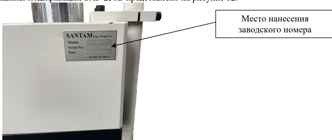
Рисунок 12 - Место нанесения заводского номера на примере машины SAF-250B
