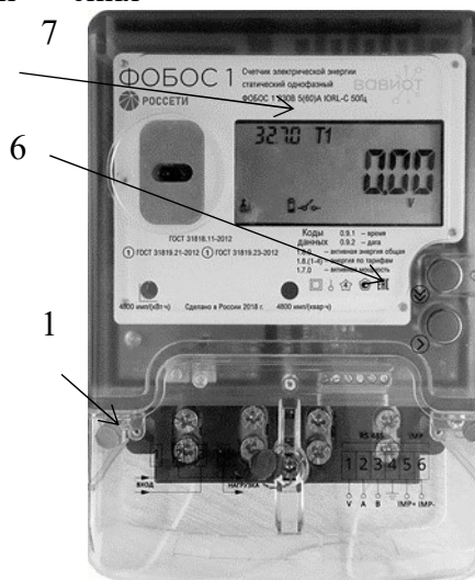
Счетчик шкафного исполнения
