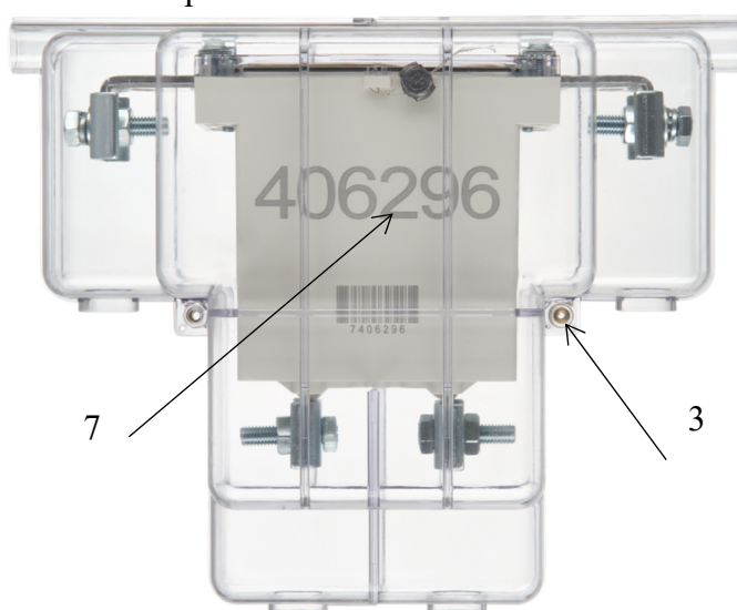
Счетчик «Базового» исполнения сплит без клеммных крышек
