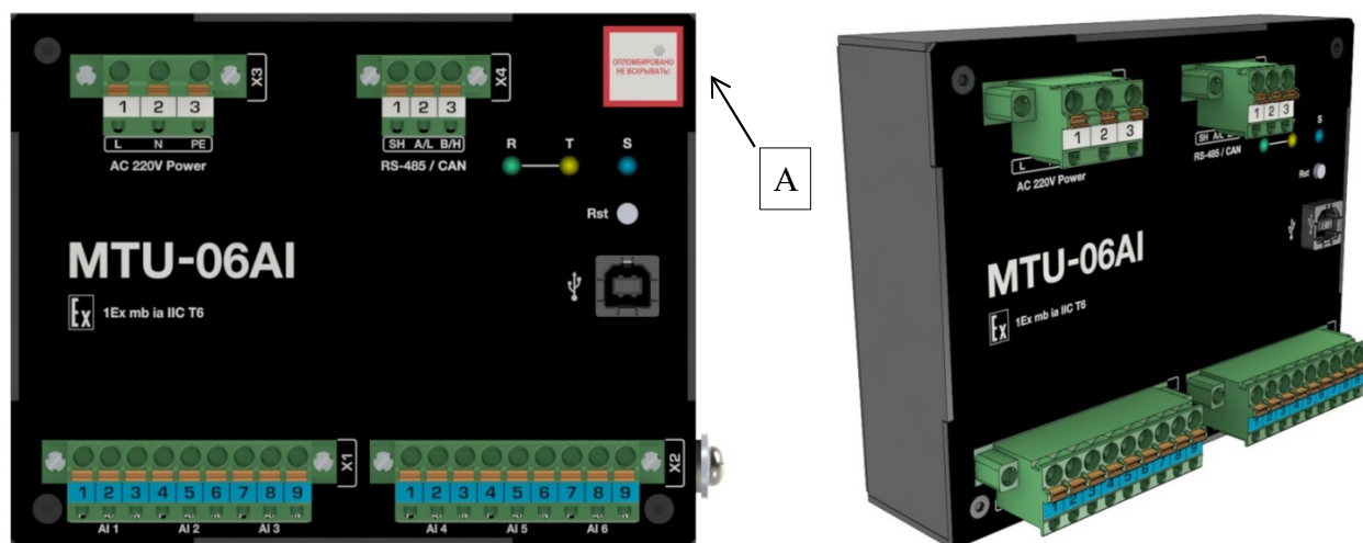
Рисунок 2 - Общий вид устройства серии MTU Место пломбировки от несанкционированного доступа (А)
