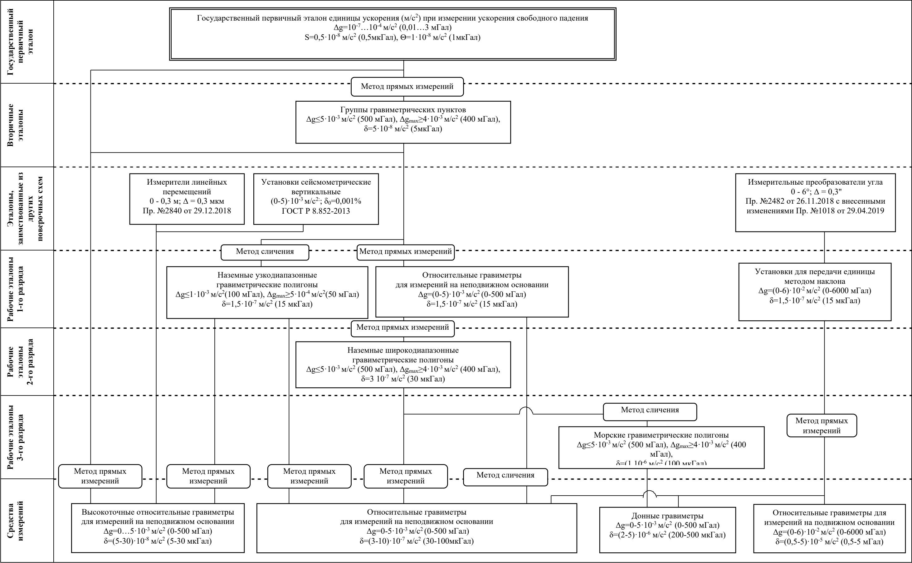
Приложение А (обязательное) А.2. Государственная поверочная схема для средств измерений ускорения свободного падения - относительная гравиметрия
