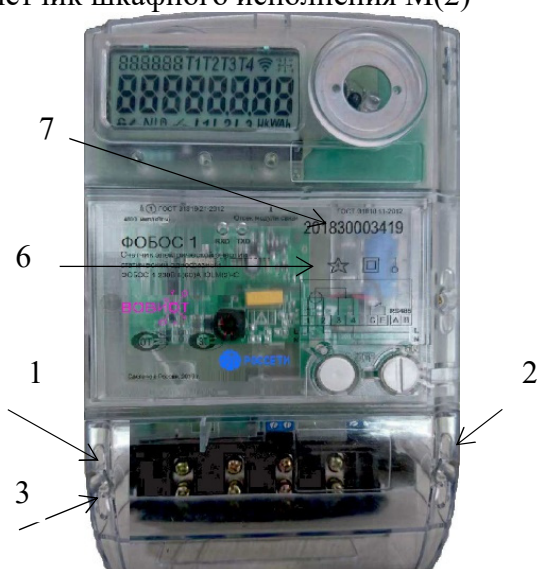
Счетчик шкафового исполнения М(2)
