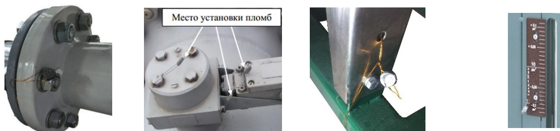
Рисунок 3 – Схемы пломбирования от несанкционированного доступа, обозначение мест нанесения знака поверки на фланцевые соединения расходомеров и/или ТПУ, детекторов ТПУ, и/или места установки (крепления) мерников к основанию (общей раме) установки, регулируемые шкалы (при наличии) мерников ( в зависимости от состава) установок поверочных автоматизированных УПРС+
