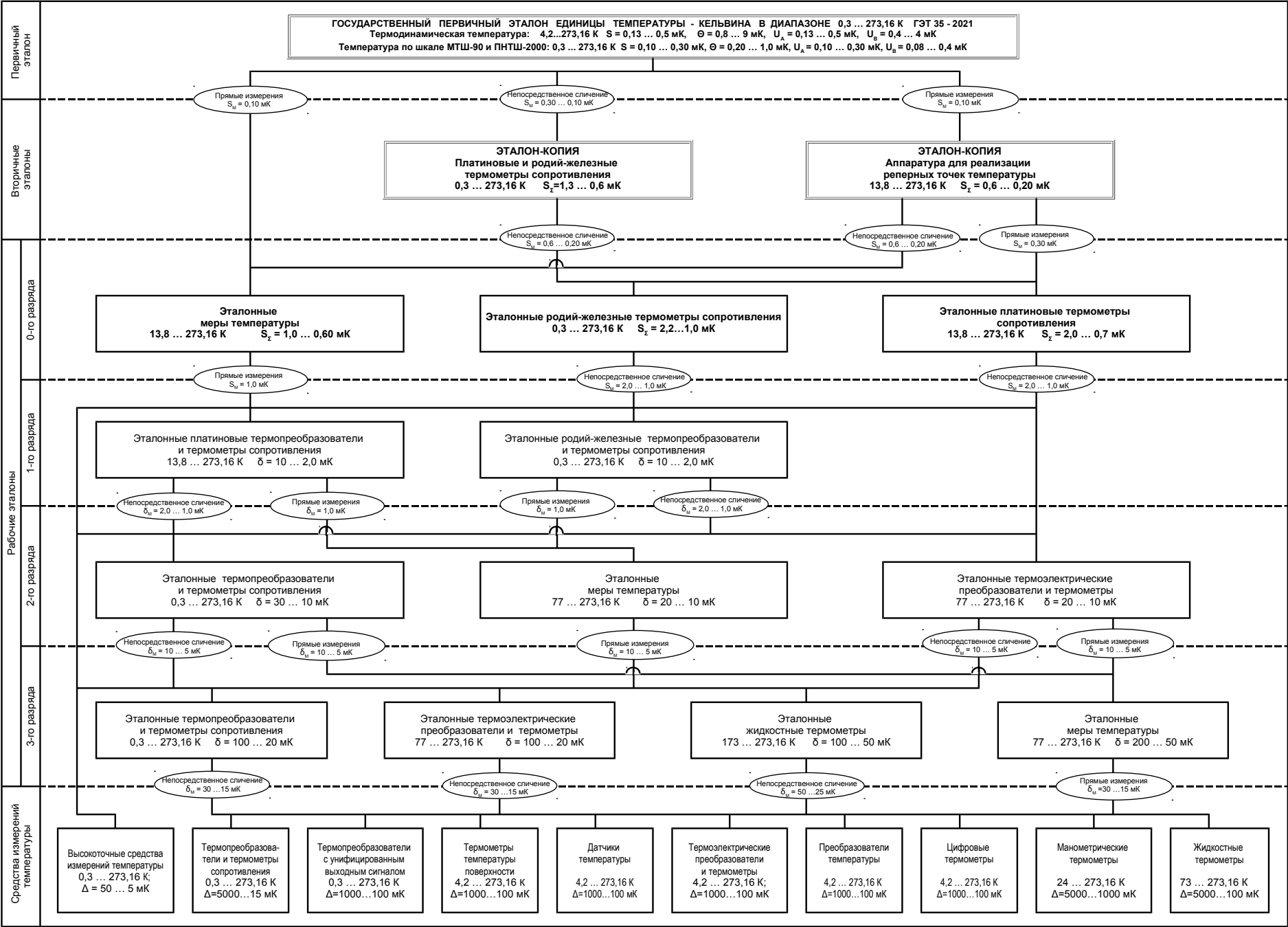
Государственная поверочная схема для контактных термометров в диапазоне температуры ниже 273,16 К (0,01 °С)
