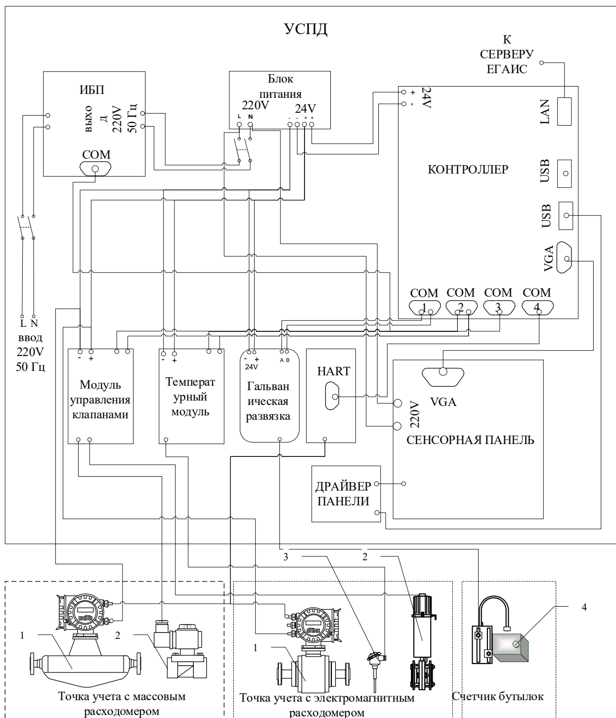
Рисунок 2 – Структурная схема комплекса 1- расходомер; 2- запорный клапан; 3- термосопротивление; 4- счетчик бутылок
