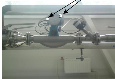
Фото 1 Расходомер Promass
