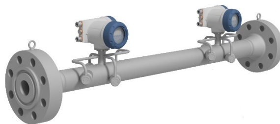
ж) OPTISONIC 4400 C/HP (редундантное исполнение)
