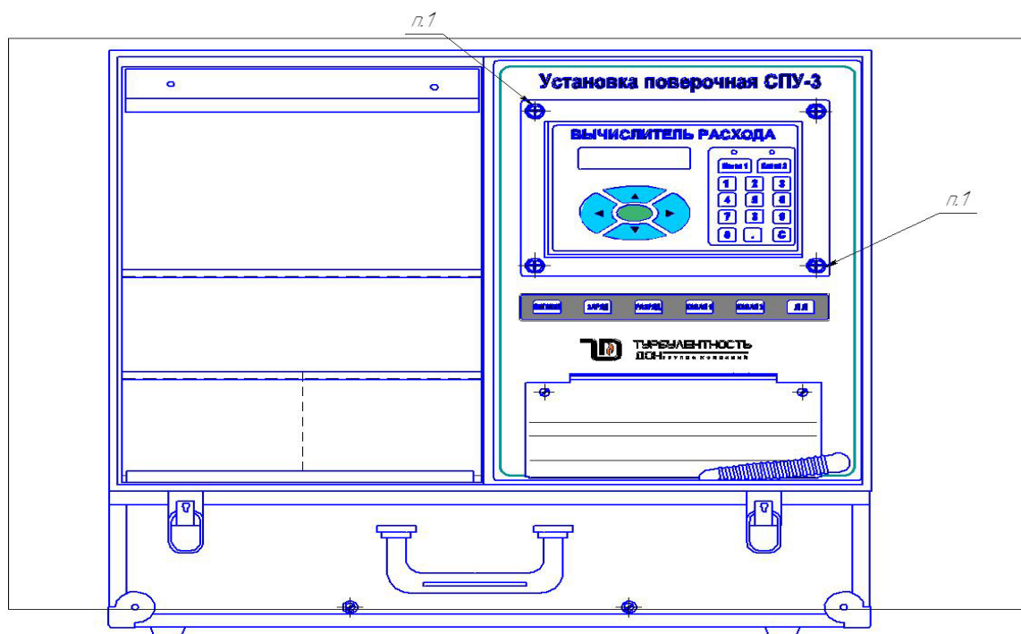
Рисунок 2 - Схема пломбирования вычислителя расхода установок
