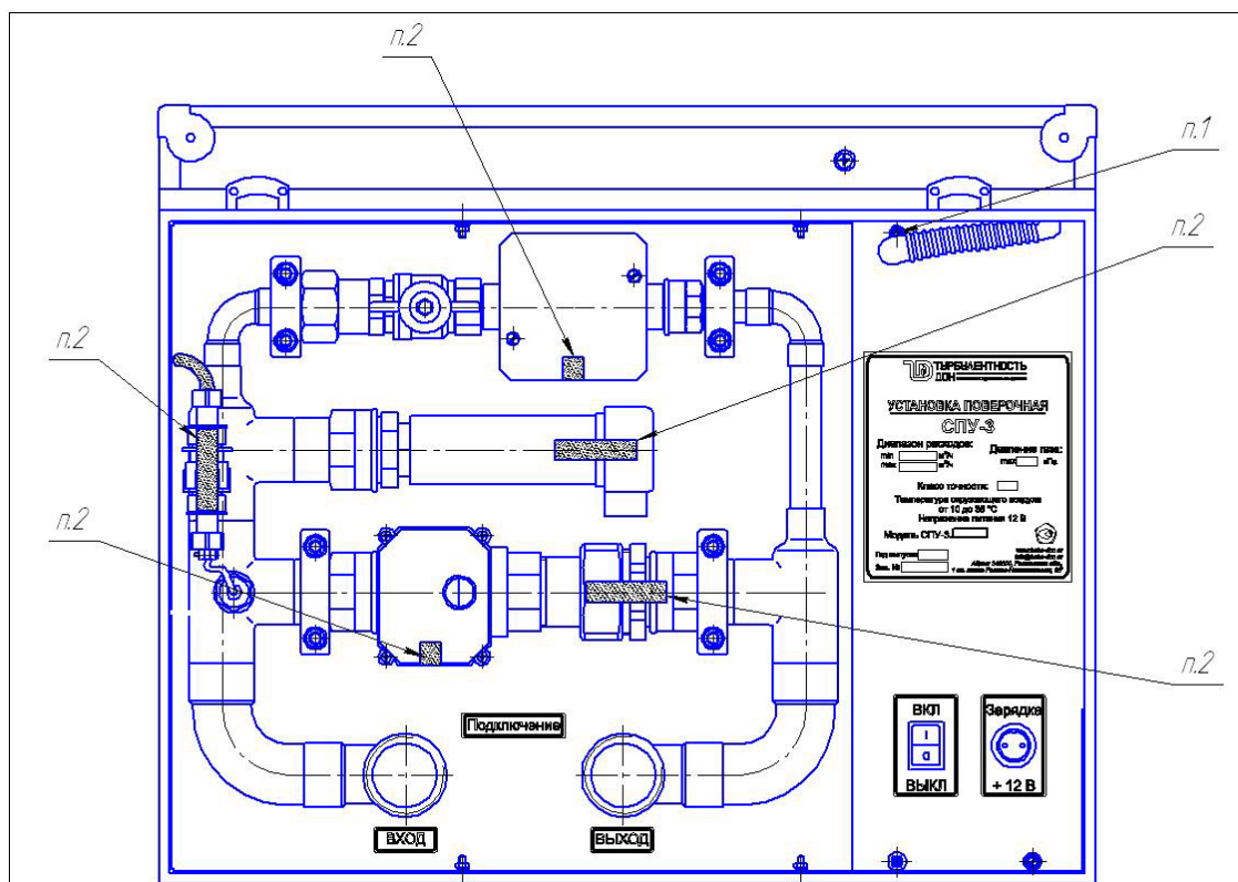
Рисунок 3 - Схема пломбирования установок
