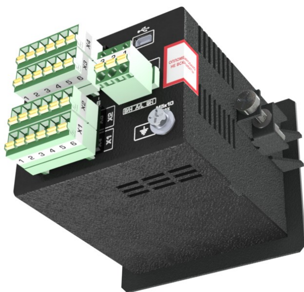
Рисунок 3 - Устройство измерения параметров нагрузки серии EM модификация 02, места нанесения пломб изготовителя Знак поверки наносится на бланк свидетельства о поверке.
