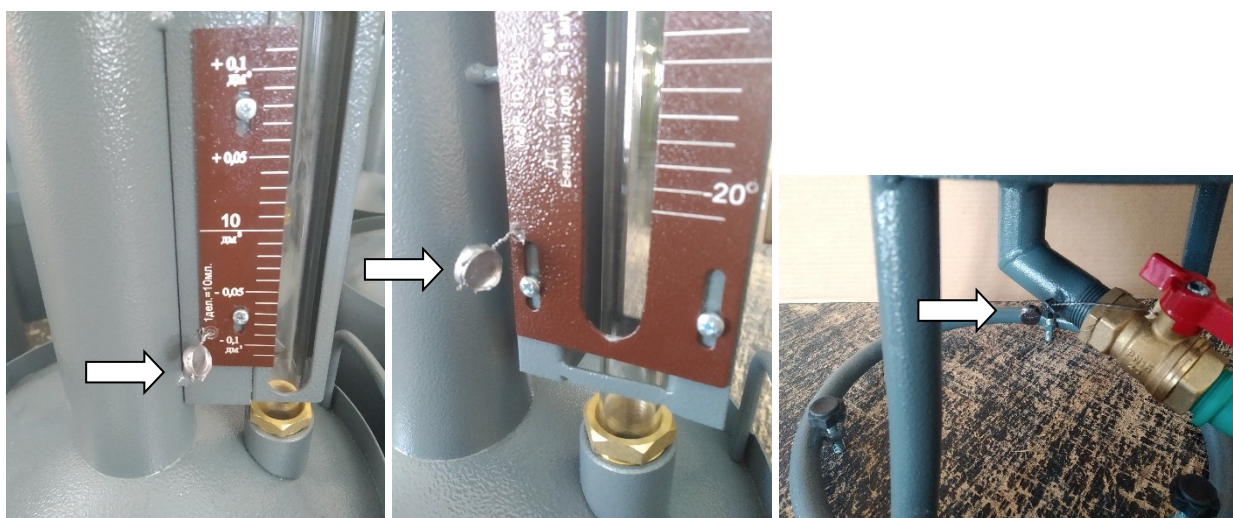
Рисунок 2 – Схема пломбировки от несанкционированного доступа, обозначение места нанесения знака поверки мерников
