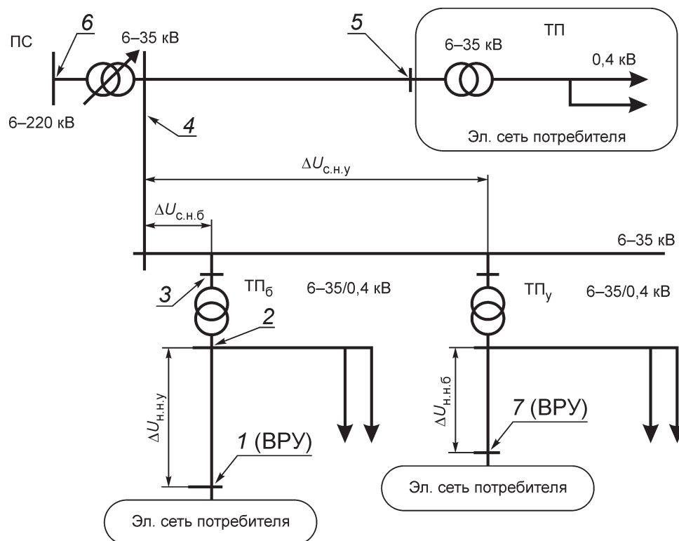
Рисунок А.1 — Схема распределительной электрической сети
