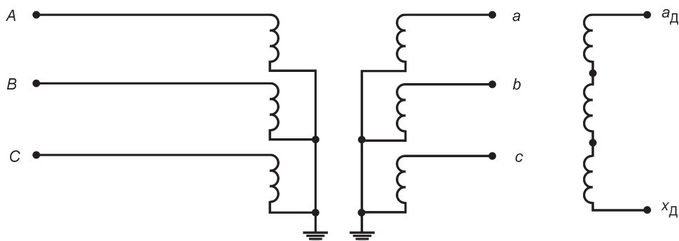
Рисунок Б.2 — Схема включения однофазных заземляемых и трехфазных заземляемых двухобмоточных трансформаторов в трехфазных сетях с изолированной нейтралью и напряжением 3—35 кВ
