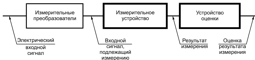
Рисунок 1 — Полная измерительная цепь
