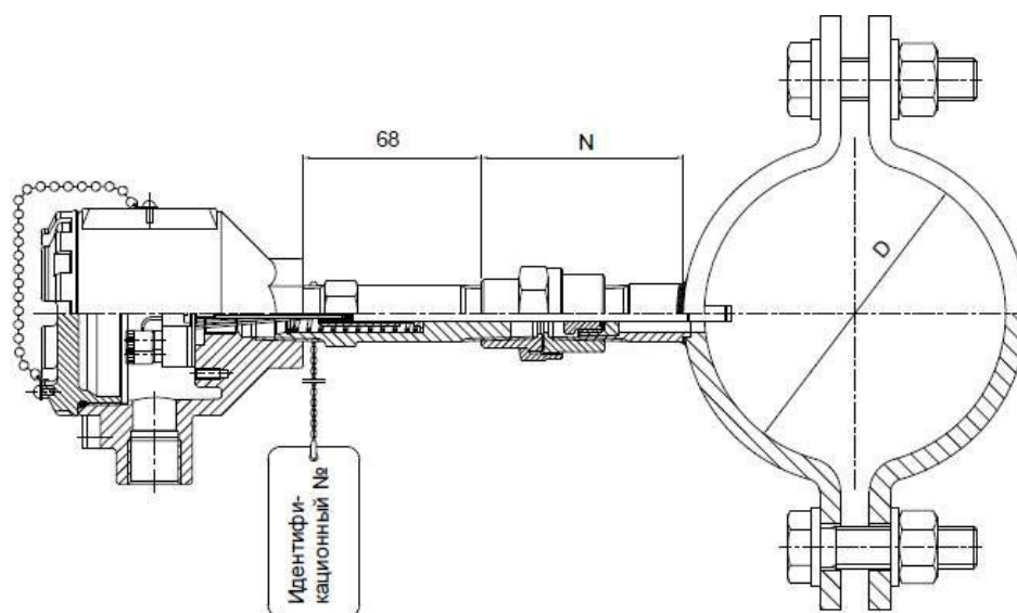
Рис.2 – ТС в сборе с монтажным хомутом
