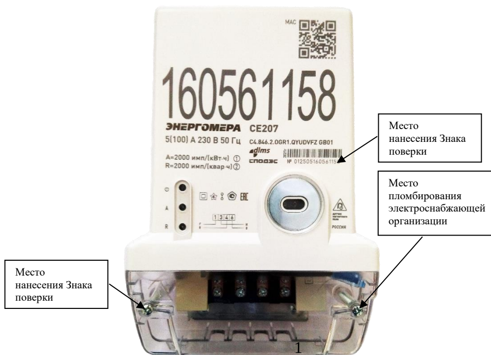
Рисунок 4 – Общий вид счетчика CE207 C4
