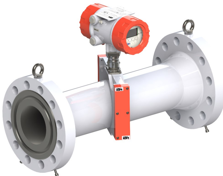
Рисунок 1в – Внешний вид счетчика в модификации КТМ600 РУС Лайт (сварной измерительный корпус)
