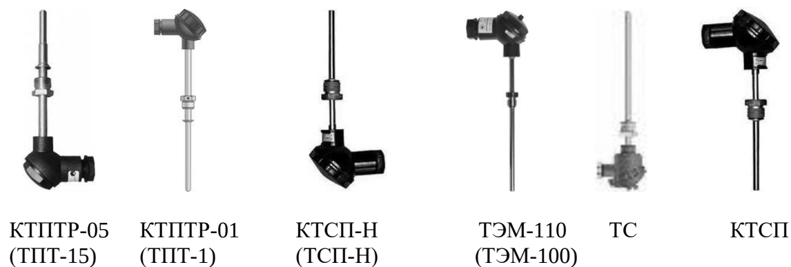
Рисунок 5 – Преобразователи температуры
