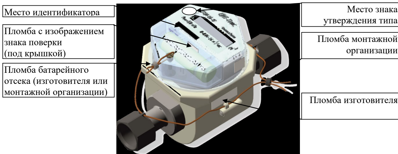
Рисунок 2 – Схема пломбирования и место нанесения знака утверждения типа
