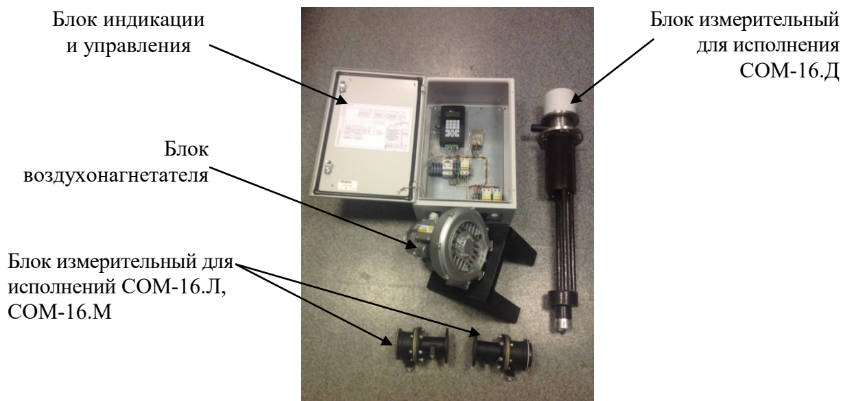
Рисунок 1 – Общий вид пылемеров СОМ-16
