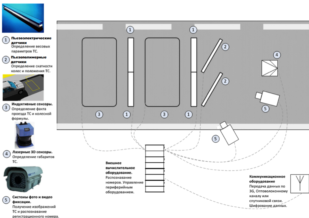
Рисунок 1 – Общий вид системы «ИБС ВИМ»
