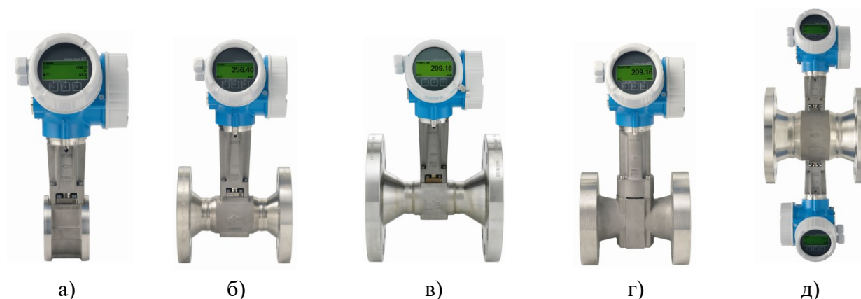
Рисунок 1. Внешний вид расходомеров Prowirl 200 в различных исполнениях: а) сенсор D; б) сенсор F; в) сенсор R; г) сенсор O; д) в исполнении Dualsens.
