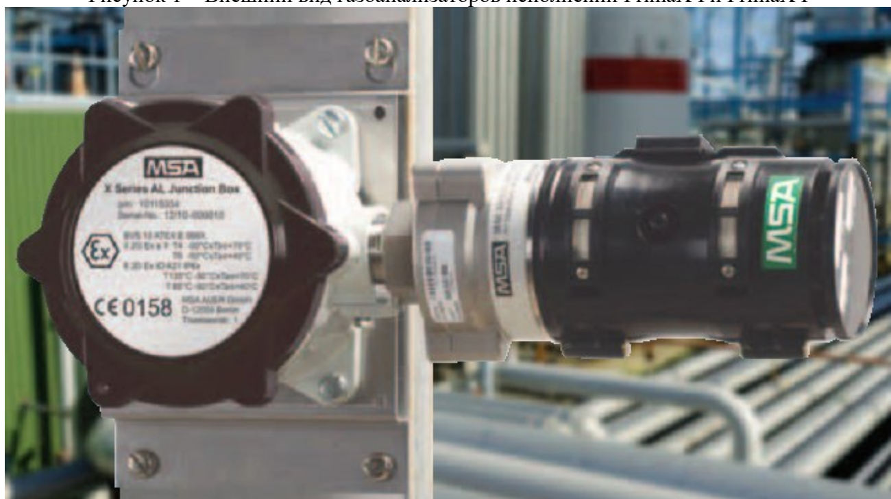
Рисунок 2 – Внешний вид газоанализаторов исполнения PrimaX IR
