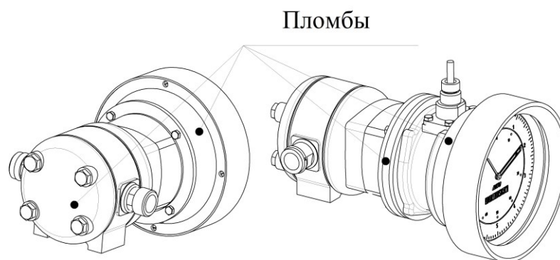
Рисунок 12 – Измеритель объема с овальными шестернями ППО. Схема пломбирования от несанкционированного доступа, обозначение мест нанесения знака поверки
