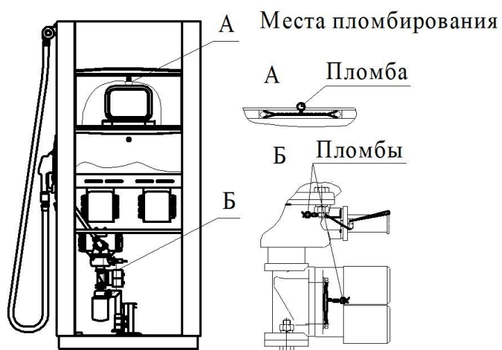
Рисунок 8 - Схема пломбирования от несанкционированного доступа, обозначение мест нанесения знака поверки
