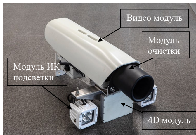
Рисунок 2 - Общий вид комплексов (видео модуль с модулями ИК подсветки, модулем очистки и 4D модулем)
